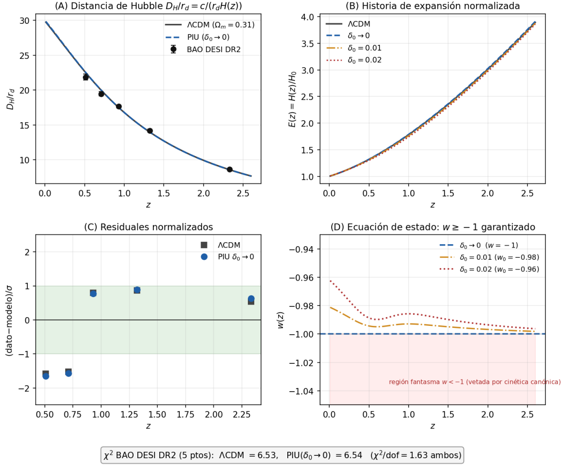
Figura 8: El fondo cósmico cuantitativo del Pleno frente a los datos. (A) La distancia de Hubble D_H/r_d = c/(r_d H(z)) del programa (PIU, \delta_0 \rightarrow 0 ) y de \Lambda\text{CDM} , comparadas con las cinco medidas BAO modelo-independientes de DESI DR2 ( z = 0,51, 0,71, 0,93, 1,32, 2,33 ); las dos curvas son indistinguibles y ajustan los puntos con \chi^2 = 6,54 frente a 6,53. (B) La historia de expansión normalizada E(z) = H(z)/H_0 : su forma es invariante de escala (ninguna escala dimensional sobrevive tras normalizar E(0) = 1 ), forzada por el potencial efectivo derivado, con la condición inicial \delta_0 como única libertad observable; al aumentar \delta_0 la curva se separa levemente de \Lambda\text{CDM} a z alto. (C) Residuales normalizados (\text{dato} - \text{modelo})/\sigma : PIU y \Lambda\text{CDM} dejan el mismo patrón, dentro de la banda de 1\sigma salvo los dos puntos de baja z que reflejan la tensión BAO-FCM que ambos modelos heredan. (D) La ecuación de estado w(z) que un observador infiere al ajustar el fondo elástico con la parametrización w_0 - w_a : aparenta w_0 > -1 hoy con un mínimo somero hacia z \approx 0,5 - 0,7 y converge a -1 , sin cruzar la frontera fantasma. La ecuación de estado del medio es w = -1 exacto (§III.7.5); la curva del panel es el artefacto de la parametrización, y el programa predice que se atenúa en observables modelo-independientes (§III.8.7). Todos los parámetros de teoría están derivados; la única libertad es la condición inicial observable \delta_0 .
