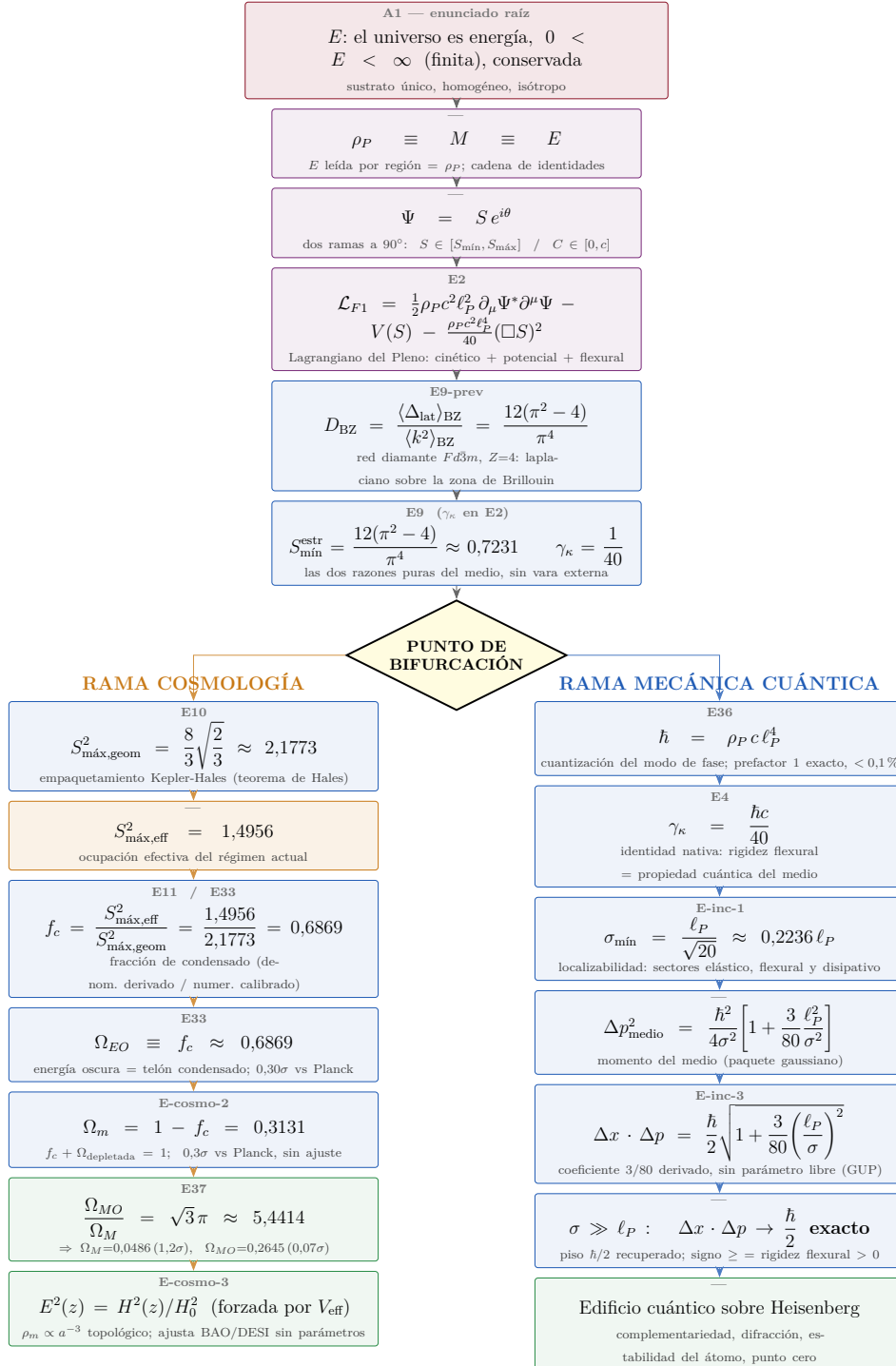
Figura 14: La cadena derivacional completa desde E . Tronco común (génesis A1→F1 y geometría de la red diamante) y bifurcación en dos ramas: a la izquierda la cosmología (hasta \Omega_m = 1 - f_c y la historia de expansión H(z) ), a la derecha la mecánica cuántica (hasta la relación de incertidumbre con piso \hbar/2 exacto). Sobre cada caja, la etiqueta de su ecuación en el manuscrito (“—” donde la expresión es una identidad sin número propio). El color del borde codifica la clasificación epistémica: tronco/fundamento , [DERIVADO] , [deducción lógica fuerte] , [CALIBRADO] . El único eslabón calibrado —el numerador S_{\text{máx,eff}}^2 — aparece marcado en su color: la rama cuántica es derivada de extremo a extremo, mientras que la cosmológica hereda un factor calibrado declarado.
