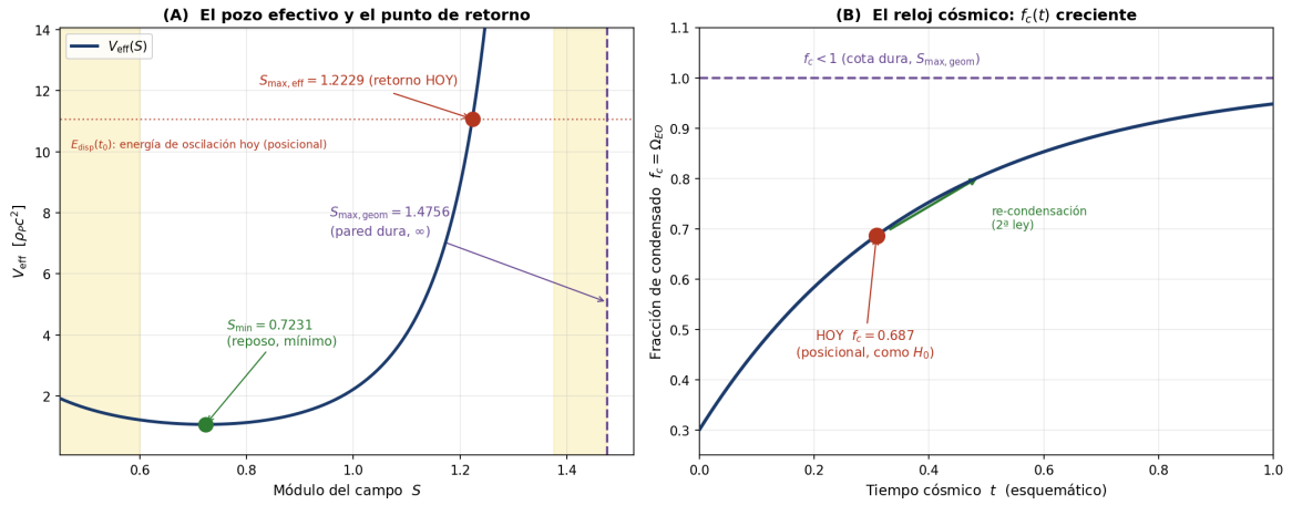
Figura 3: La fracción de condensado f_c = \Omega_{EO} como posición en una trayectoria, no como constante. (A) El módulo del Pleno-suelo oscila en el pozo efectivo V_{\text{eff}} (forma cerrada derivada, E11-bis) entre la pared cuántica IR ( V_q = 3\rho_{\text{PC}}^2/8S^2 ) y la pared de Gent UV; reposa en el mínimo S_{\text{min}}^{\text{estr}} = 0,7231 [DERIVADO] y su excursión máxima actual alcanza el punto de retorno S_{\text{máx,eff}} = 1,2229 (al cuadrado, 1,4956), fijado por la energía de oscilación disponible hoy E_{\text{disp}}(t_0) = 10,003 \rho_{\text{PC}}^2 —cantidad posicional, análoga a H_0 , no una constante derivable. El eje horizontal es el módulo S ; las etiquetas S_{\text{máx,geom}} = 1,4756 y S_{\text{máx,eff}} = 1,2229 son las raíces de las cotas, mientras que la fracción f_c y la comparación física se leen siempre en S^2 . (B) La fracción de condensado f_c está acotada por la cota dura f_c < 1 ; el valor presente f_c = 0,687 es la posición del reloj cósmico hoy, no un número fundamental. El estatus [CALIBRADO] del numerador S_{\text{máx,eff}}^2 es, por tanto, la marca correcta de un valor de estado posicional, no una debilidad provisional.
