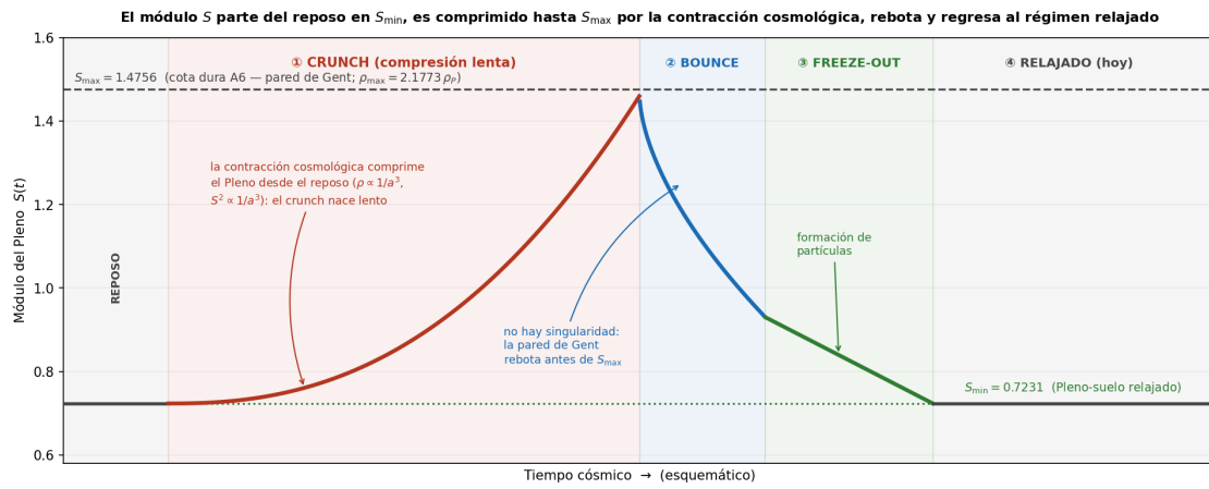
Figura 5: La cronología cosmológica del Pleno como un ciclo crunch-bounce completo. El módulo parte del reposo en el Pleno-suelo ( S_{\min} = 0,7231 ) y es comprimido por la contracción cosmológica ( \rho_{\text{medio}} = \rho_P S^2 , \rho \propto 1/a^3 ): el crunch nace lento desde el fondo y acelera hacia S_{\max} . Antes de alcanzar la cota dura A6, la pared de Gent detiene el colapso y produce el bounce —un rebote finito, sin singularidad, en lugar del Big Bang singular de la Relatividad General. Sigue el freeze-out (congelamiento de constantes y formación de partículas) y el regreso al régimen relajado actual en S_{\min} . El ciclo es asimétrico (volumen creciente entre ciclos); nuestro universo observable es la fase posterior al último bounce.
