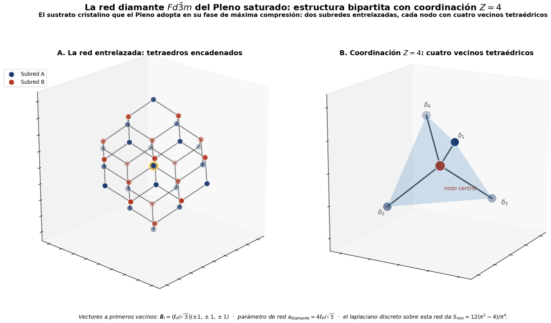
Figura 2: La red diamante Fd\bar{3}m que el Pleno adopta en su fase saturada. (A) Celda convencional: la estructura consta de dos subredes FCC entrelazadas (A en azul, B en rojo), desplazadas un cuarto de la diagonal del cubo —esta bipartición A/B es la que sostiene el sector de fase y la neutralidad cósmica. (B) El motivo de coordinación Z = 4 : cada nodo tiene exactamente cuatro vecinos en disposición tetraédrica, conectados por los vectores \delta_i = (\ell_P/\sqrt{3})(\pm 1, \pm 1, \pm 1) . La coordinación 4 es el mínimo que satisface el criterio de isostaticidad de Maxwell en 3D, una de las cuatro razones convergentes que justifican esta geometría. El promedio espectral del laplaciano discreto sobre esta red produce la forma cerrada S_{\min} = 12(\pi^2 - 4)/\pi^4 .
