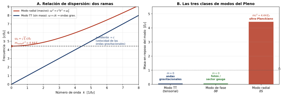
Figura 4: El espectro de modos del Pleno. (A) Relación de dispersión: el modo radial \delta S es masivo (rama con gap \omega_0 = \sqrt{\xi} c/\ell_P , masa m_{\text{radial}} c^2 = 4.44 E_P ), mientras que el modo TT no tiene gap y propaga a velocidad c —las ondas gravitacionales. (B) Las tres clases de modos según su masa-en-reposo: el modo TT (ondas gravitacionales) y el modo de fase (fotón/sector gauge) son ambos sin masa y constituyen los observables del programa; el modo radial es ultra-Planckiano ( 4.44 E_P ), lo que explica por qué el Pleno no se detecta como partícula. El gap del modo radial sale de la curvatura del potencial, \xi = V''_{\text{eff}}(S_{\text{mín}})/(\rho_P c^2) = 19.69 . El valor 4.44 E_P es la masa elástica (tree-level, rigidez estática del pozo); la resolución completa de la relación de dispersión da además una masa propagante de 3.50 E_P (gap de la rama física tras la regulación flexural). Ambas son ultra-Planckianas; la distinción es ontológica, sin consecuencia observacional (§III.1.9).
