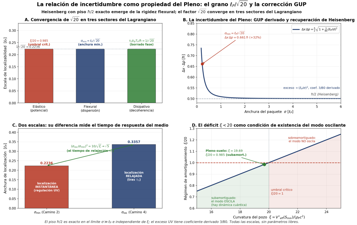
Figura 6: La relación de incertidumbre como propiedad estructural del Pleno. (A) El factor \sqrt{20} converge en tres sectores físicamente distintos del Lagrangiano —elástico (umbral de amortiguamiento \xi/20 ), flexural (anchura mínima \sigma_{\min} = \ell_P/\sqrt{20} ) y disipativo (borrado de fase \tau_{\Pi} k_B T_P / \hbar = 1/\sqrt{20} )—, definiendo una escala de localizabilidad genuina del medio, \ell_P/\sqrt{20} \approx 0,2236 \ell_P . (B) La relación de incertidumbre del Pleno, \Delta x \Delta p = (\hbar/2) \sqrt{1 + (3/80)(\ell_P/\sigma)^2} (E-inc-3): recupera el piso \hbar/2 exacto para \sigma \gg \ell_P y predice un exceso ultravioleta (GUP) con coeficiente derivado 3/80; en \sigma = \sigma_{\min} el producto vale 0,661 \hbar (exceso del 32%). (C) Las dos escalas de localización —instantánea \sigma_{\min} (Camino 2) y relajada \sigma_{\text{osc}} (Camino 4)— no se contradicen: su cociente (\sigma_{\text{osc}}/\sigma_{\min})^2 = 10/\sqrt{\xi} \rightarrow \sqrt{5} es el factor del tiempo de relajación \tau_{\Pi} , de modo que la diferencia entre ambas mide el tiempo de respuesta del medio. (D) El déficit \xi = 19,69 < 20 no es imperfección sino condición de existencia: solo del lado subamortiguado ( \xi/20 < 1 ) el modo radial oscila y sostiene la dinámica cuántica; el Pleno está sintonizado tan cerca del umbral crítico como puede sin apagar la oscilación. Todas las escalas, sin parámetros libres.
