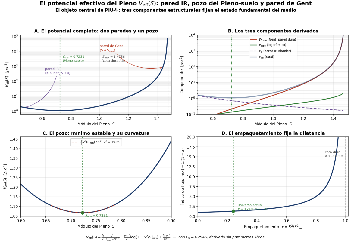
Figura 1: El potencial efectivo V_{\text{eff}}(S) , objeto central de PIU- \Psi . (A) El potencial completo en escala logarítmica: la pared cuántica IR de Klauder impide S \rightarrow 0 , el pozo fija el Pleno-suelo en S_{\text{mín}} = 0,7231 , y la pared de Gent impide S \rightarrow S_{\text{máx}} = 1,4756 (cota dura A6). (B) Descomposición en los tres componentes derivados: W_{\text{bare}} (Gent), V_{\text{topo}} (logarítmico) y V_q (pared IR). (C) Zoom del pozo, con la parábola de curvatura V''(S_{\text{mín}}) = 19,69 \rho_P c^2 que confirma el mínimo estable. (D) El empaquetamiento x = S^2/S_{\text{máx}}^2 fija el índice de flujo dilatante n(x) = 1/(1-x) ; el universo actual está en x = 0,240 , n = 1,32 (casi newtoniano). Todos los parámetros derivados sin ajuste.
