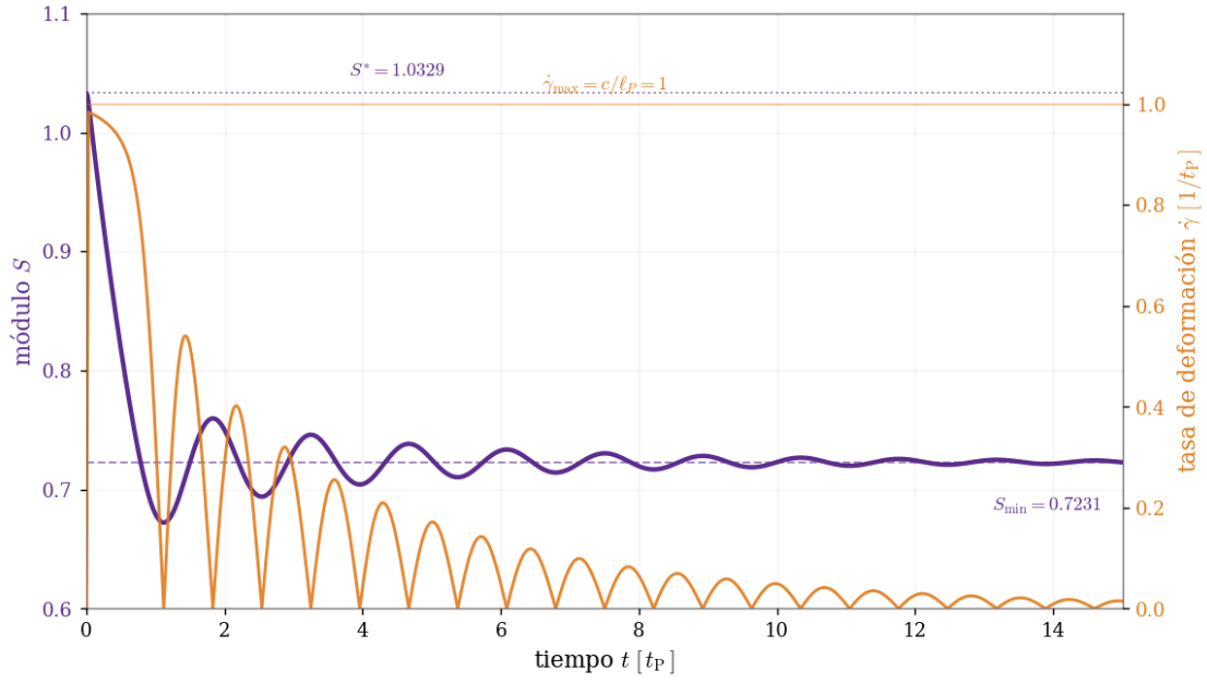
Figura 12: Trayectoria del módulo durante el transitorio de cristalización , integrando la ecuación de movimiento viscosa con todos los coeficientes derivados. El módulo S(t) (violeta, eje izquierdo) desciende monótono de S^* = 1,033 y sobrepasa S_{\min} por inercia hasta un mínimo absoluto de 0,672 en t \approx 1,1 t_P , tras lo cual oscila con amplitud decreciente y se asienta en S_{\min} = 0,7231 . La tasa de deformación \dot{\gamma}(t) (naranja, eje derecho) alcanza un máximo de 0,98 —rozando la cota de Planck \dot{\gamma}_{\max} = c/\ell_P = 1 sin superarla— durante la bajada rápida, y pulsa hacia cero en cada punto de retorno del módulo (donde \dot{S} = 0 ). Los picos decrecientes de \dot{\gamma} son la firma del amortiguamiento viscoso. El tiempo está en tics de Planck.
