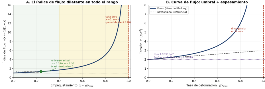
El Pleno como fluido dilatante de Herschel-Bulkley: índice de flujo y curva reológica
