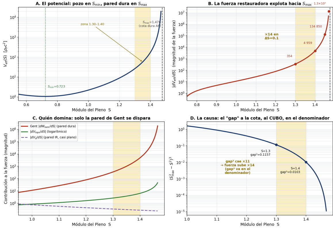
Figura 10: La pared de Gent del Pleno. (A) El potencial V_{\text{eff}}(S) : pozo en S_{\min} , pared dura en S_{\max} . (B) La fuerza restauradora |dV_{\text{eff}}/dS| en escala logarítmica, explotando hacia S_{\max} ; marcados los valores de la zona discutida. (C) Descomposición en los tres términos: solo la pared de Gent (rojo) se dispara; V_{\text{topo}} y V_q quedan muy por debajo. (D) La causa raíz: el gap (S_{\max}^2 - S^2)^3 en el denominador, que cae \times 11 entre S = 1,30 y S = 1,40 y dispara la fuerza \times 14 .
