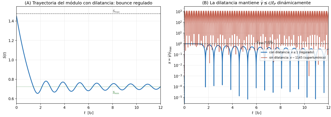
Figura 11: Integración numérica de la ecuación del ciclo (E57). (A) Trayectoria del módulo S(t) con la viscosidad dilatante: el bounce está regulado y el módulo oscila entre S_{\min} y la compresión inicial sin alcanzar S_{\max} . (B) Tasa de deformación x = \dot{\gamma}/\dot{\gamma}_{\max} : con dilatancia (azul) se mantiene acotada por la cota x \leq 1 —la viscosidad diverge en x = 1 y frena el bounce antes de cruzarla; sin el mecanismo dilatante (rojo, amortiguamiento constante) la tasa escala hasta \sim 1,1 \times 10^3 \dot{\gamma}_{\max} , tres órdenes de magnitud sobre la cota, físicamente imposible. La dilatancia es el regulador que mantiene el bounce subluminal. Integración con scipy (método Radau, tolerancias 10^{-9}/10^{-11} , convergencia verificada bajo refinamiento del paso); parámetros todos derivados ( E_0 = 4,2546 , S_{\max} = 1,4756 , S_{\min} = 0,7231 , \eta_0 = 0,1027 ).
